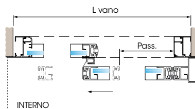
Sezione Orizzontale ASD 1+1, Profilo 32 mm
