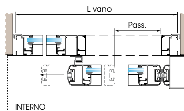
Sezione Orizzontale ASD 1+1, Profilo 50 mm
