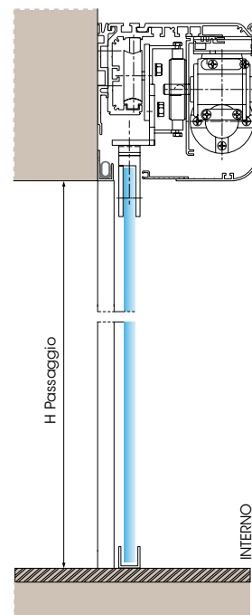
Sezione Verticale GLAZED 2 A Soluzione con ante tutto vetro temperato o stratificato 10 mm
