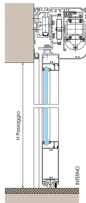
Sezione Verticale porta ASD2 Profilato Ponzi serie 50 mm Vetro stratificato pvb 0,76 mm
