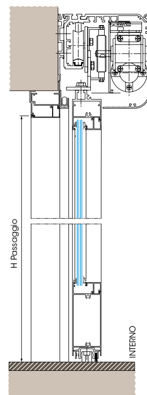
Sezione Verticale porta ASD4 Profilato Ponzi serie 50 mm Vetro stratificato pvb 0,76 mm
