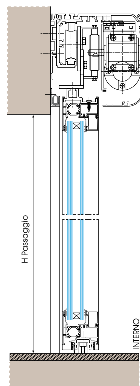
Sezione Verticale porta T.T. Profilo Taglio Termico 62 mm Vetro isolante di ampio spessore
