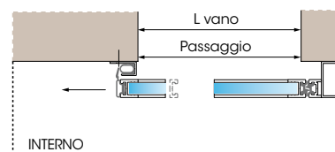
Sezione Orizzontale ASD 1, Profilo 20 mm
