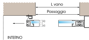
Sezione Orizzontale ASD 1, Profilo 32 mm
