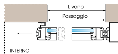
Sezione Orizzontale ASD 1, Profilo 50 mm
