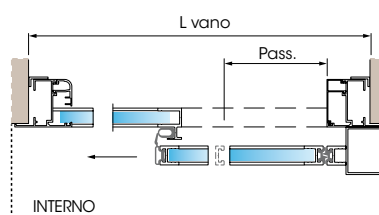
Sezione Orizzontale ASD 1+1, Profilo 20 mm
